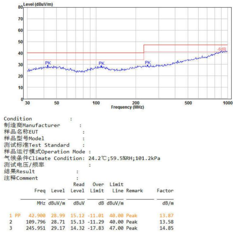
图 7-7 辐射测试垂直方向
