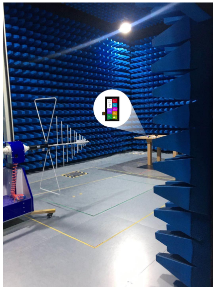
图 7-5 辐射测试图
