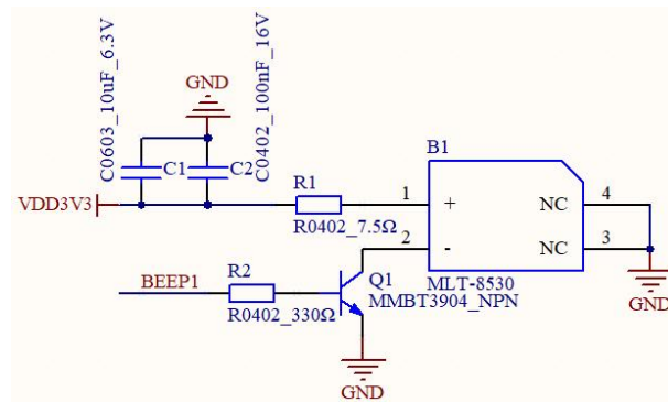
图 6-4 蜂鸣器参考电路
