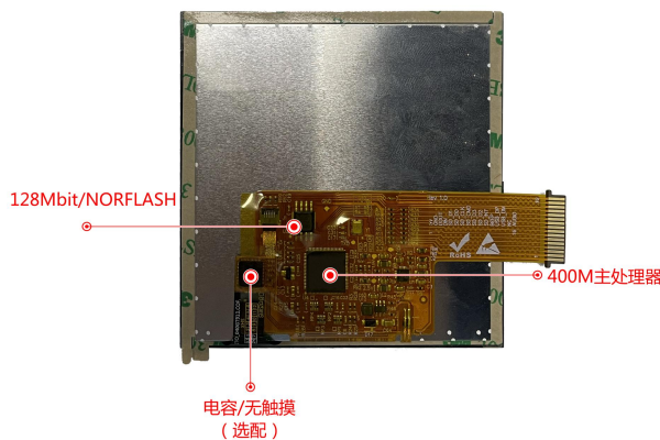
图 1-3 硬件配置图
