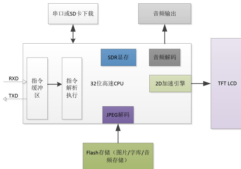
图 12-1 M 系列串口屏内部结构图
