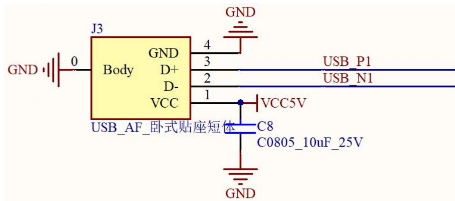
图 6-5 U 盘参考电路
