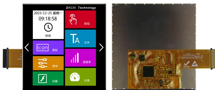
图 1-2 4.0 寸无触摸参考图
